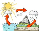
Vattnets kretslopp
